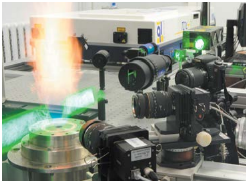
Диагностика горения в факеле с закрученного потока
