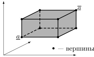
Рис. 1. Интервальный вектор \mathbf{a} = [\underline{a}, \bar{\mathbf{a}}] в \mathbb{R}^3 , его вершины, нижняя грань \underline{a} = (\underline{a}_1, \underline{a}_2, \underline{a}_3) и верхняя грань \bar{\mathbf{a}} = (\bar{a}_1, \bar{a}_2, \bar{a}_3) .
