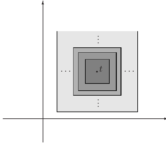
Рис. 2. Объединение кубиков с общим центром.
