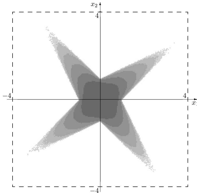
Рис. 3. Эмпирическая плотность вероятности на множестве решений интервальной линейной системы Барта — Нудинга и оптимальные по координатам оценки множества решений.
