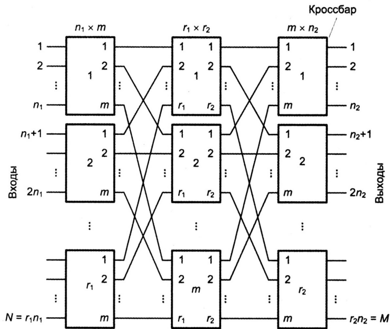
Трехступенчатая сеть с топологией Клоза
