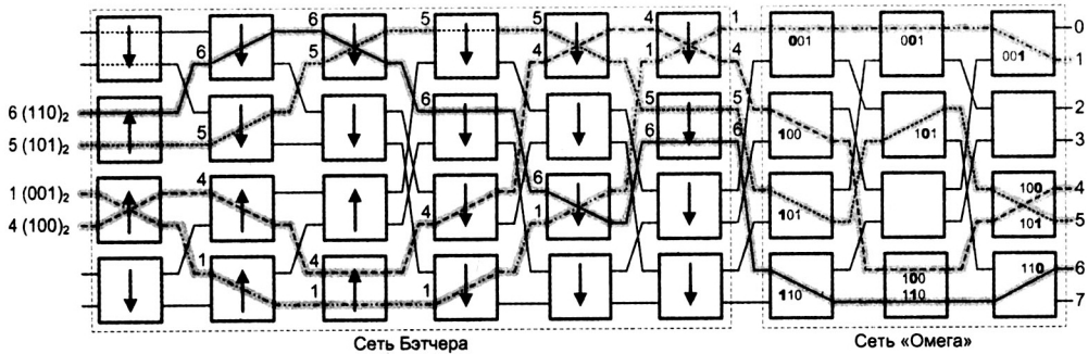
Сеть Бэтчера-Баньяна
